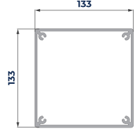
Dikme Profili Pole Profile
