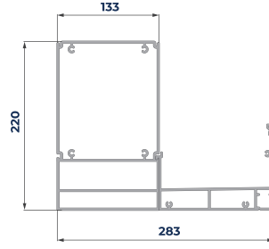
Kiriş & Oluk Profili Beam & Groove Profile
